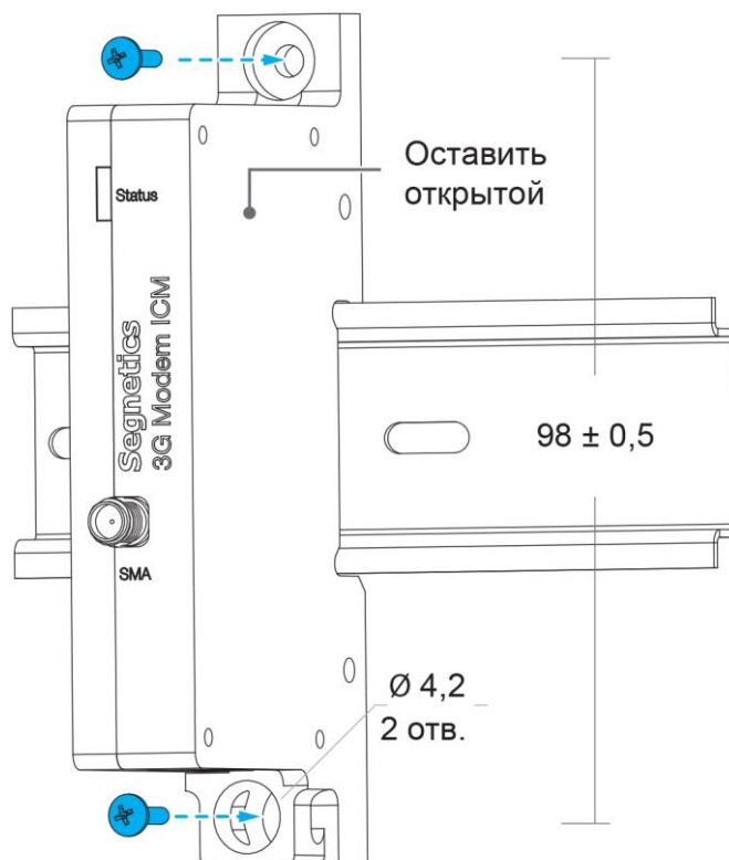
Рис. 8 – Монтаж на DIN-рейку
