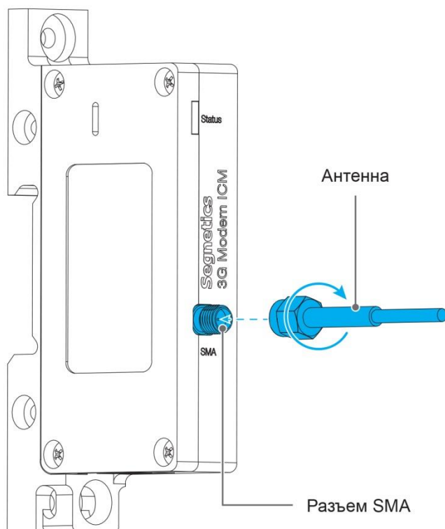
Рис. 9 – Подключение антенны
